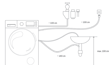
Правосторонний патрубок
