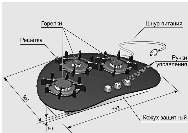
Рис. 1 МОДЕЛЬ СН2120
