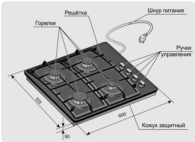
Рис. 2 МОДЕЛЬ СВН2230; -01
