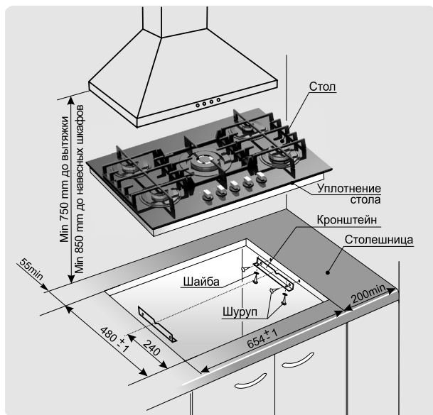
Рис. 6 МОДЕЛЬ CH2340
