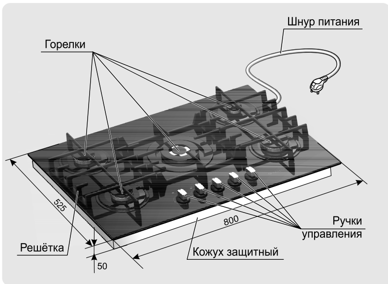
Рис. 3 МОДЕЛЬ СН2340
